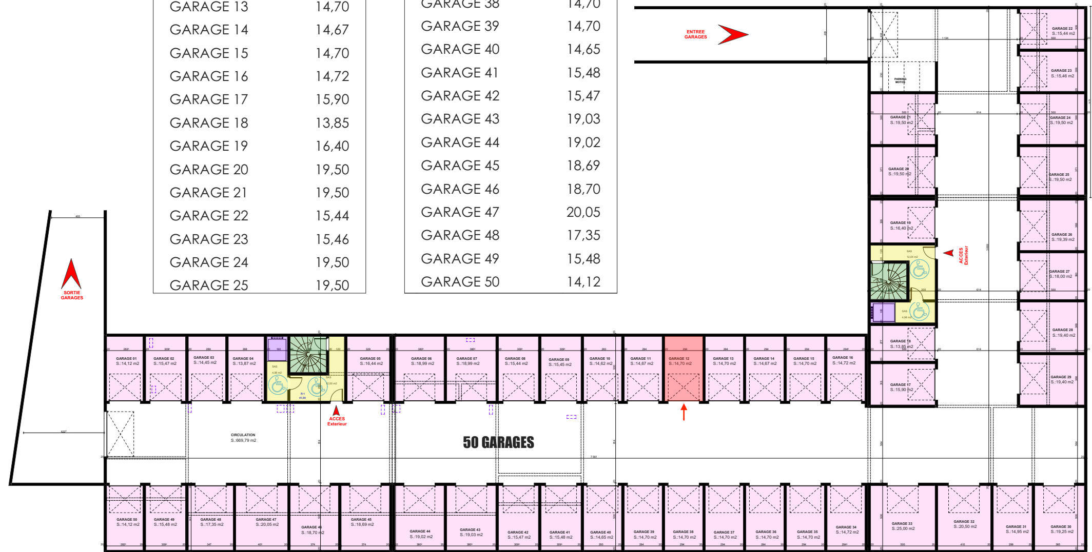
Plan d'étage courant R-1
