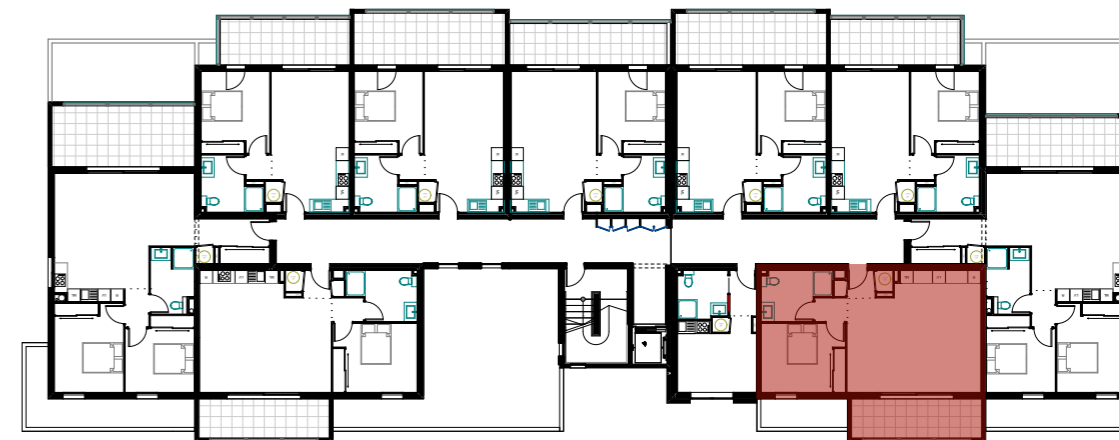
Plan d'étage courant R+1
